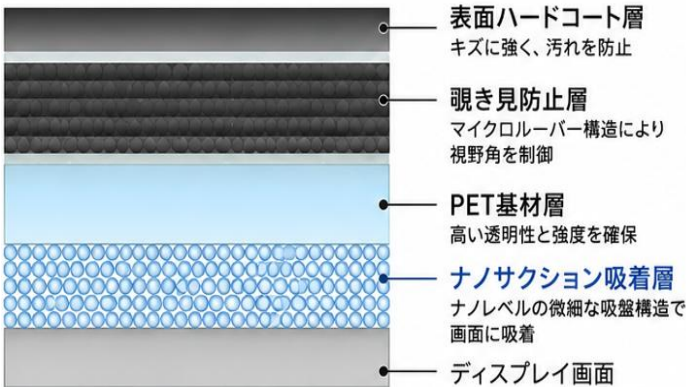
断面構造図（イメージ）
